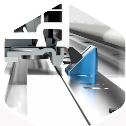
ПЛАСТИКОВЫЙ КОМПЕНСАТОР ФАЛЕВОЙ ЗАЩЕЛКИ ДЛЯ БЕСШУМНОГО И МЯГКОГО ЗАКРЫВАНИЯ
