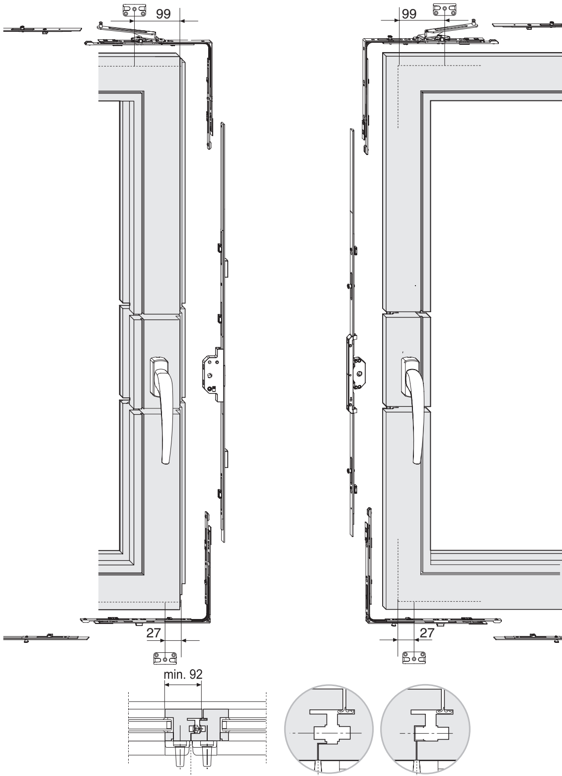
Ohne Pfosten
