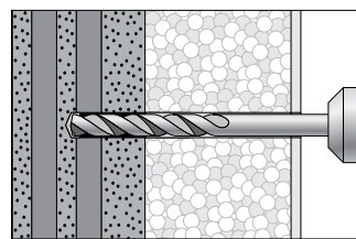
1. Bohrloch herstellen.*
