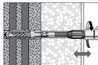
5. Beschlägeträger einschrauben und justieren.
