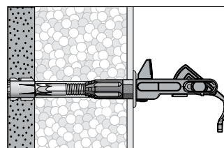
9. Montare il fermapersiana.
