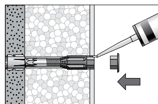
6. Sigillare contro la pioggia e montare il tappo di copertura.
