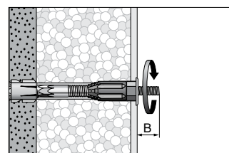
8. Gewindeschraube montieren und handfest anziehen.
