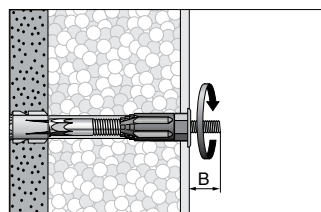
8. Montare la vite e stringerla.
