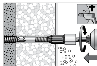
2. Putz aufräsen.
