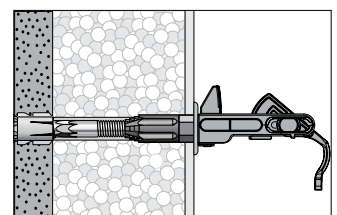
9. Ladenhalter montieren.
