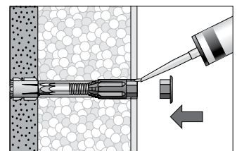
6. Schlagregenfest abdichten und Abdeckkappen aufstecken.
