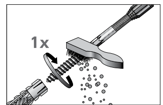
3. Beschlägeträger reinigen. Kunststoffdübel ca. eine Umdrehung auf Beschlägeträger drehen.
