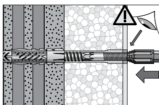
4. Inserire l'unità nel foro, finché il taglio termico è a filo intonaco.
