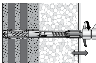
5. Avvitare e registrare il perno portante.
