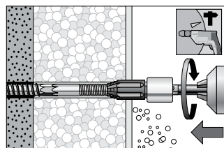
2. Fresare l'intonaco.
