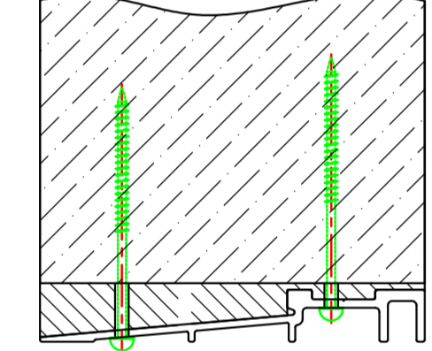
Variante 1 Fissaggio inferiore con viti
