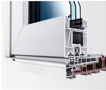
ONDERCONSTRUCTIE "ISOLATIEPROFIEL"
