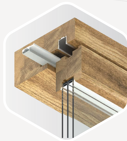
DICHTINGSPROFIEL Vlak – voor extra comfort
