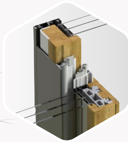
MITTELDICHTSCHIENE
