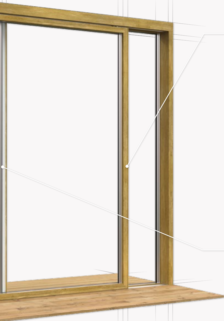
VERSTÄRKUNGSPROFIL Aus glasfaserverstärktem Kunststoffkern
