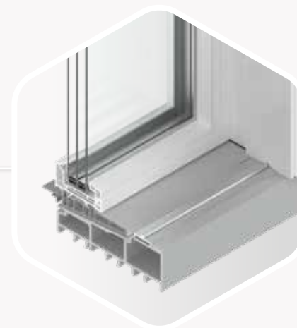
ПОРОГ С глухим остеклением: для изготовления широкоформатных конструкций с большой площадью остекления
