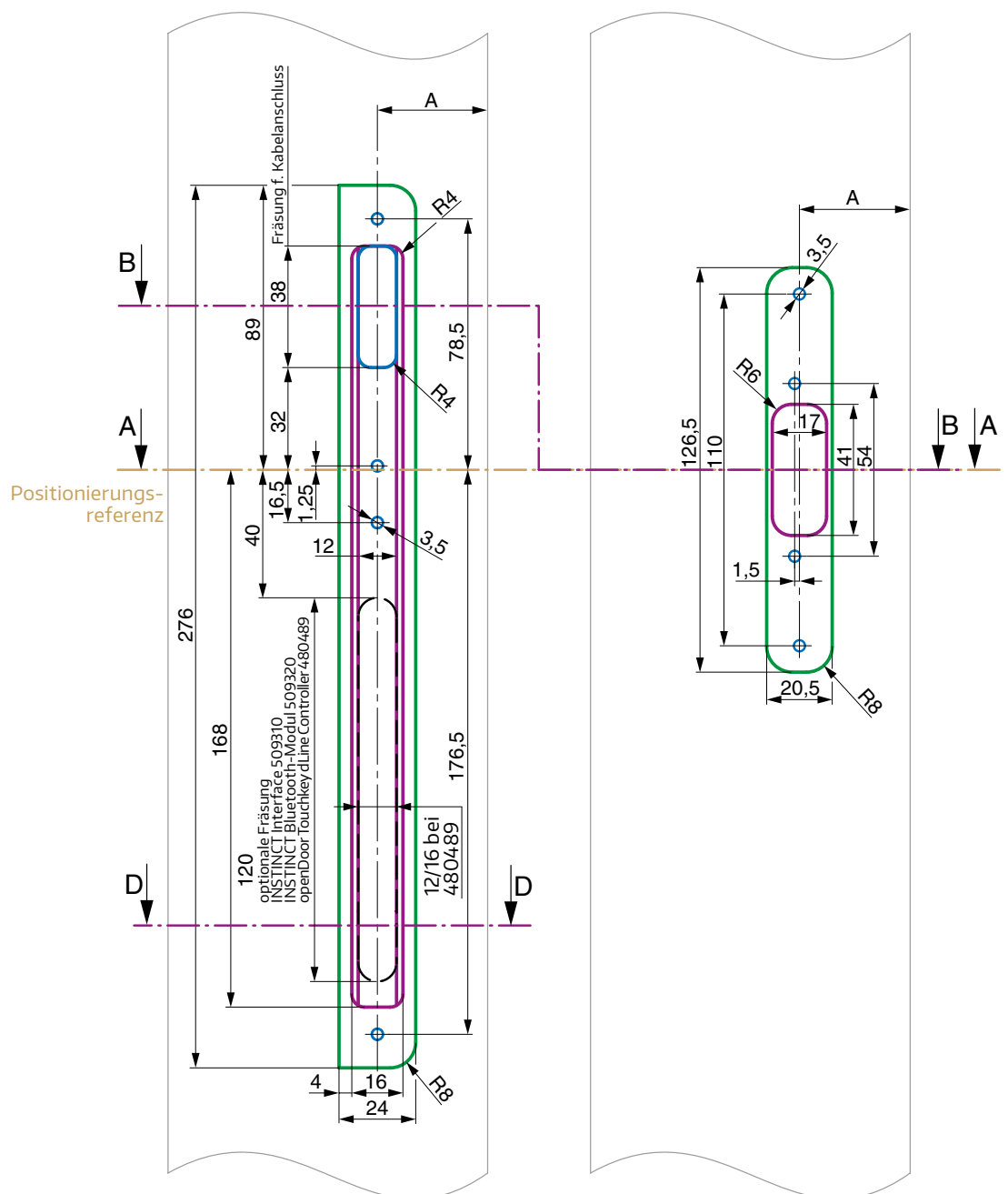
Rahmenprofil (vereinfachte Darstellung)
