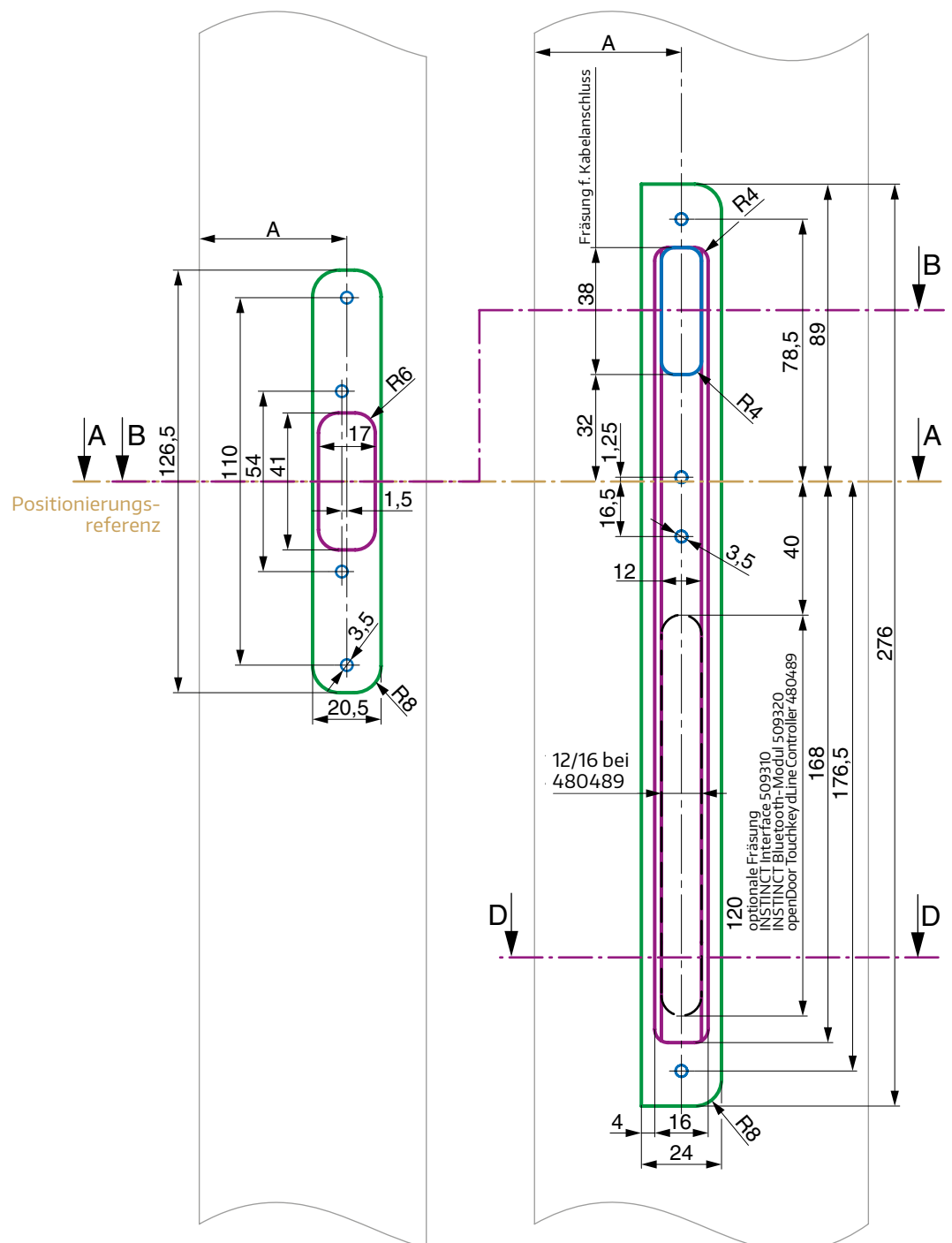
Rahmenprofil (vereinfachte Darstellung)
