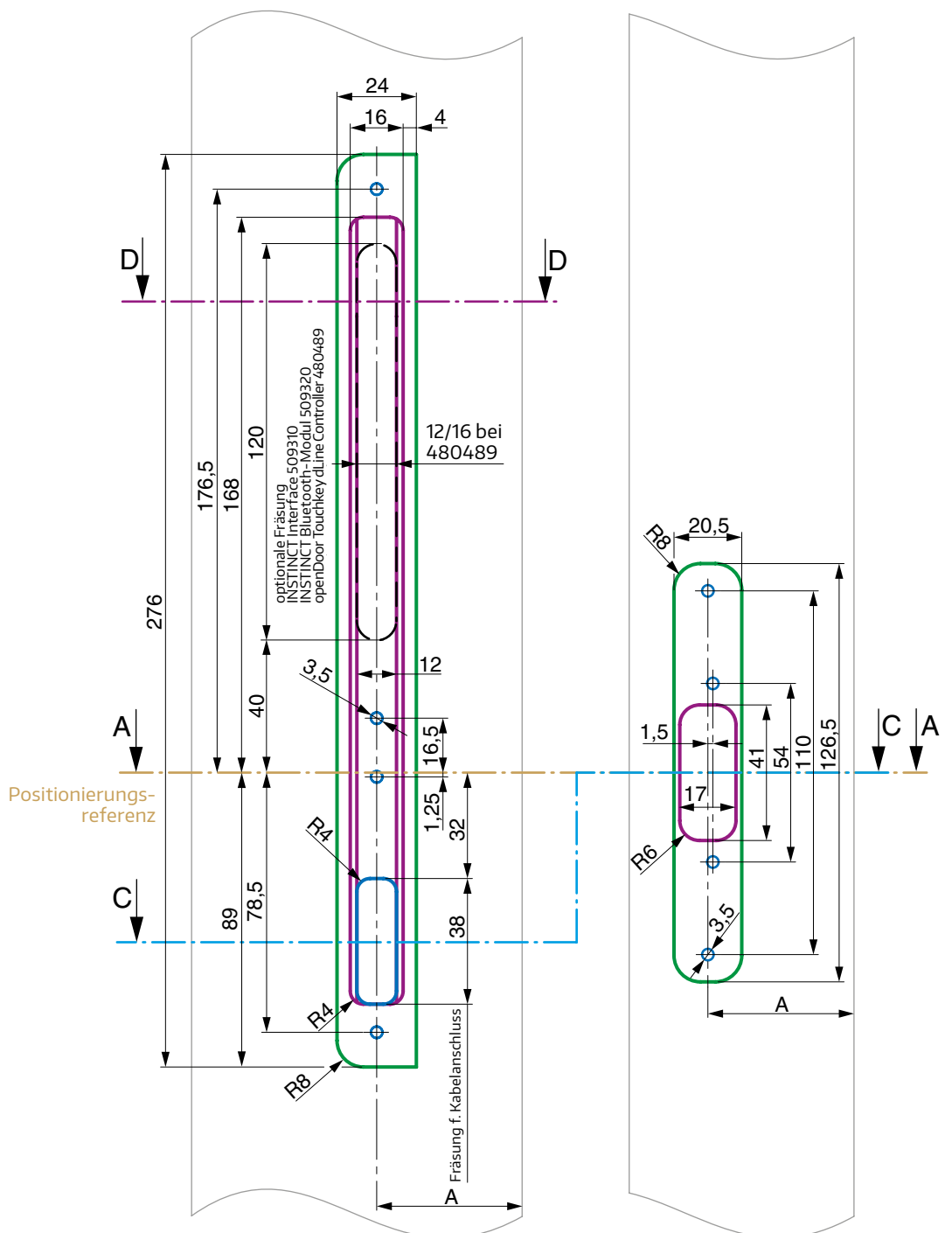
Flügelprofil (vereinfachte Darstellung)
