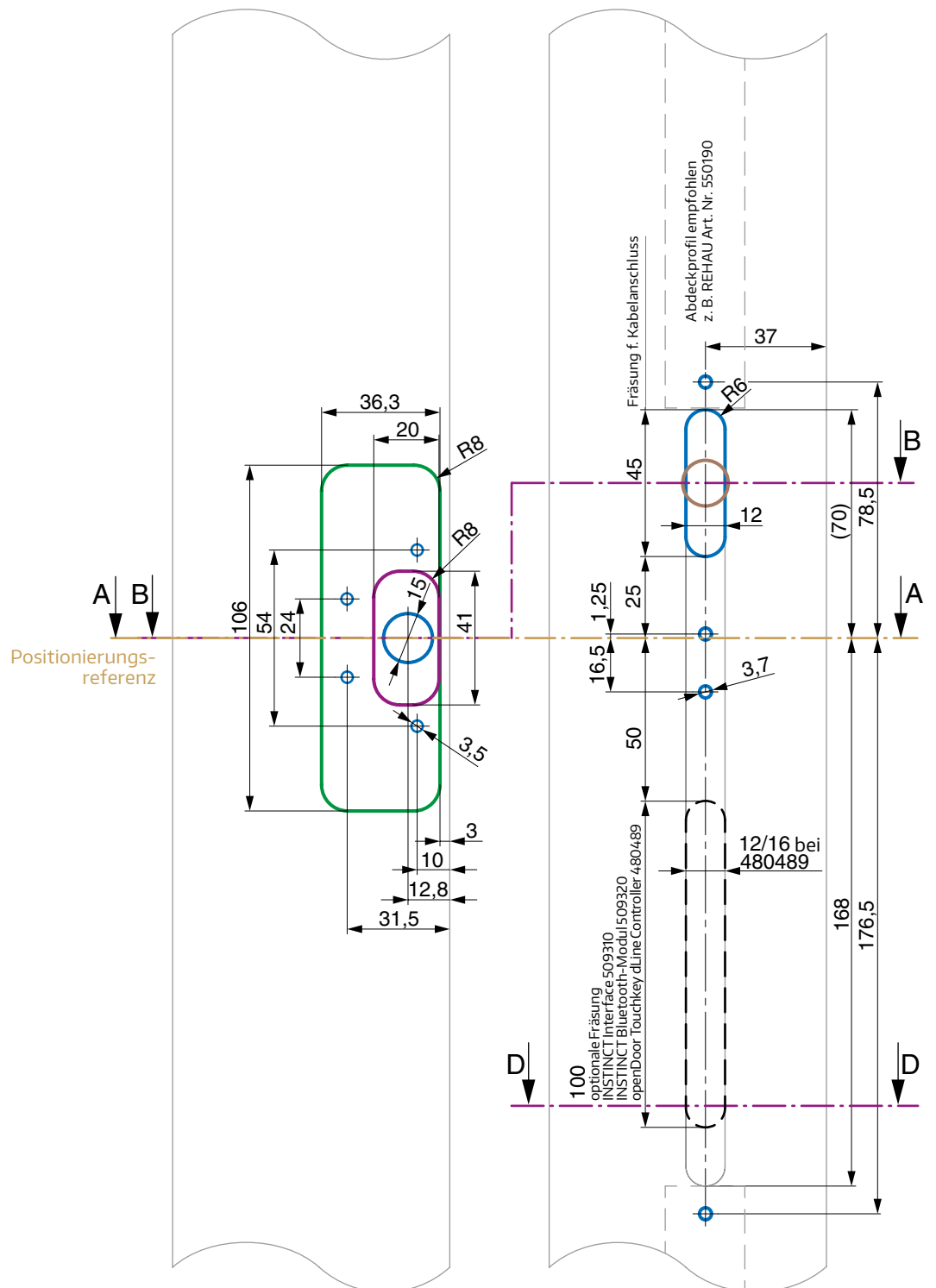
Rahmenprofil (vereinfachte Darstellung)
