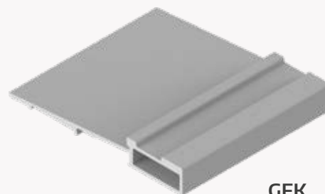
GFK 212 / 29 mm
