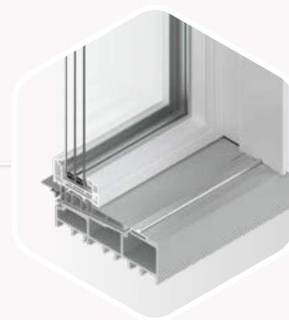
SEUIL STRUCTURÉ Vitrage fixe : pour réaliser de grandes surfaces vitrées
