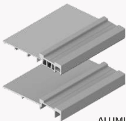
ALUMINIUM avec rupture de pont thermique ou GFK 164 / 25 mm
