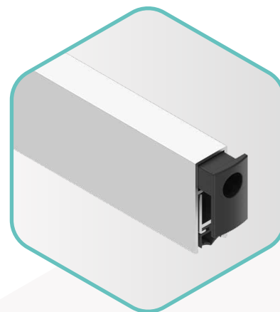
Samoregulirajuća padajuća podna brtva za vrata
