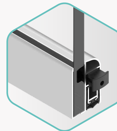
Onderdeurdichting glas
