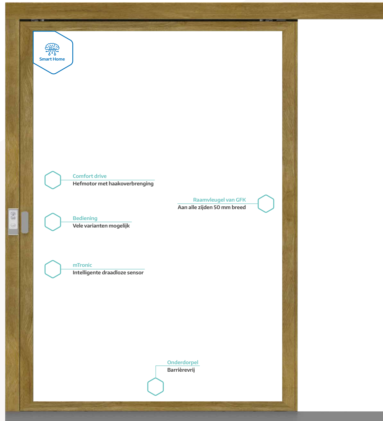
Hef-schuifdeur schema A gemotoriseerd (binnen hout, buiten aluminium)
