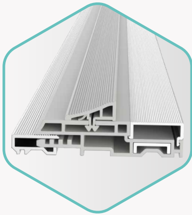
Onderdorpel Transit Personal voor vleugelafdichting
