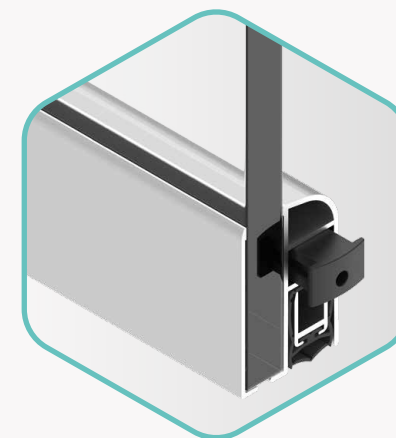
Podlahové tesnenie pre sklenené dvere
