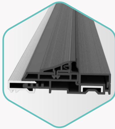
Umbral Transit Personal para junta en marco
