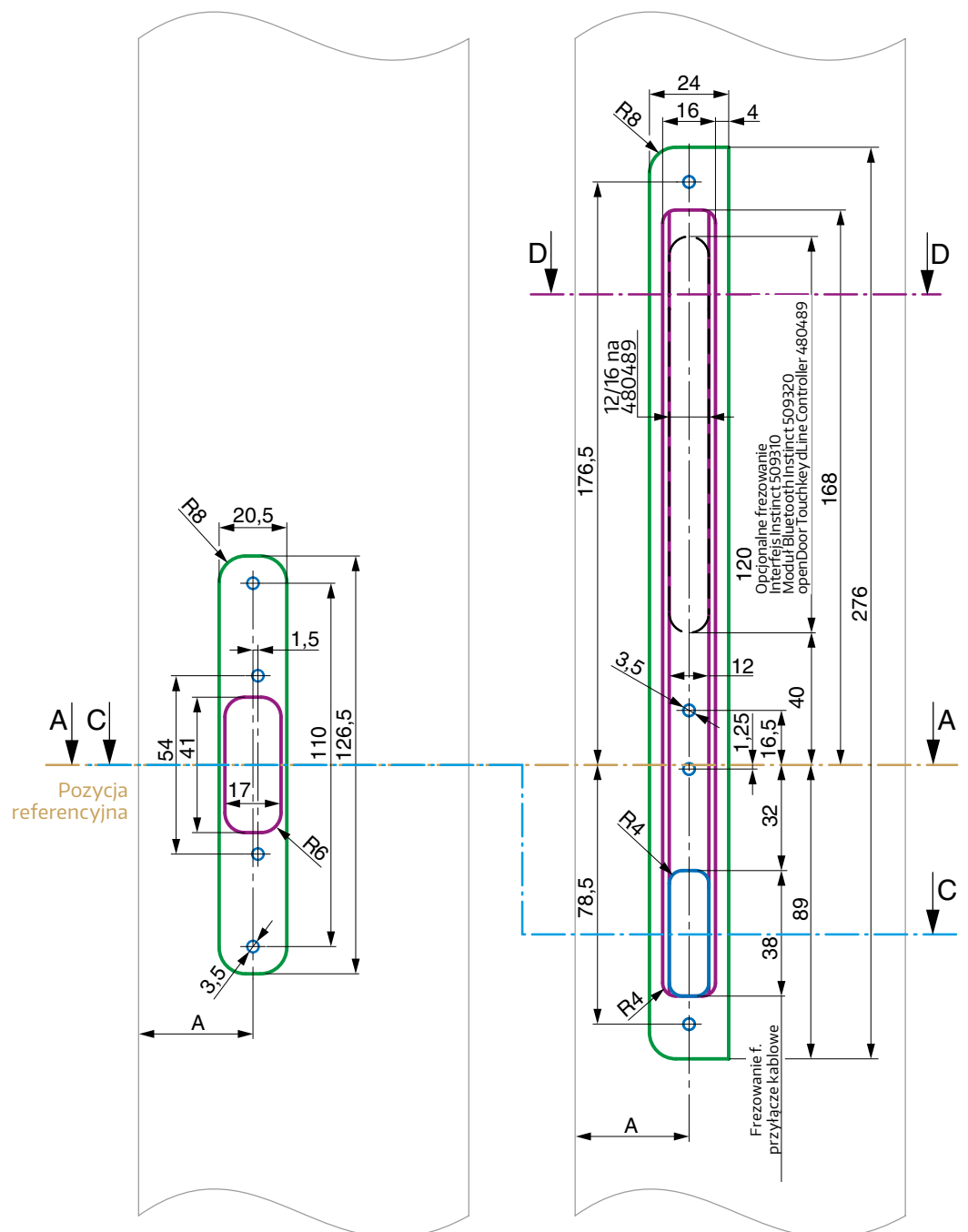
Profil skrzydła (przedstawienie uproszczone)
