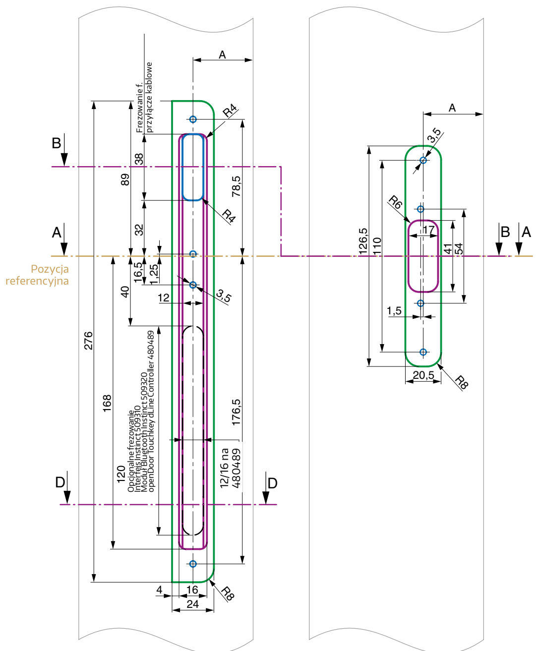
Profil ościeżnicy (przedstawienie uproszczone)
