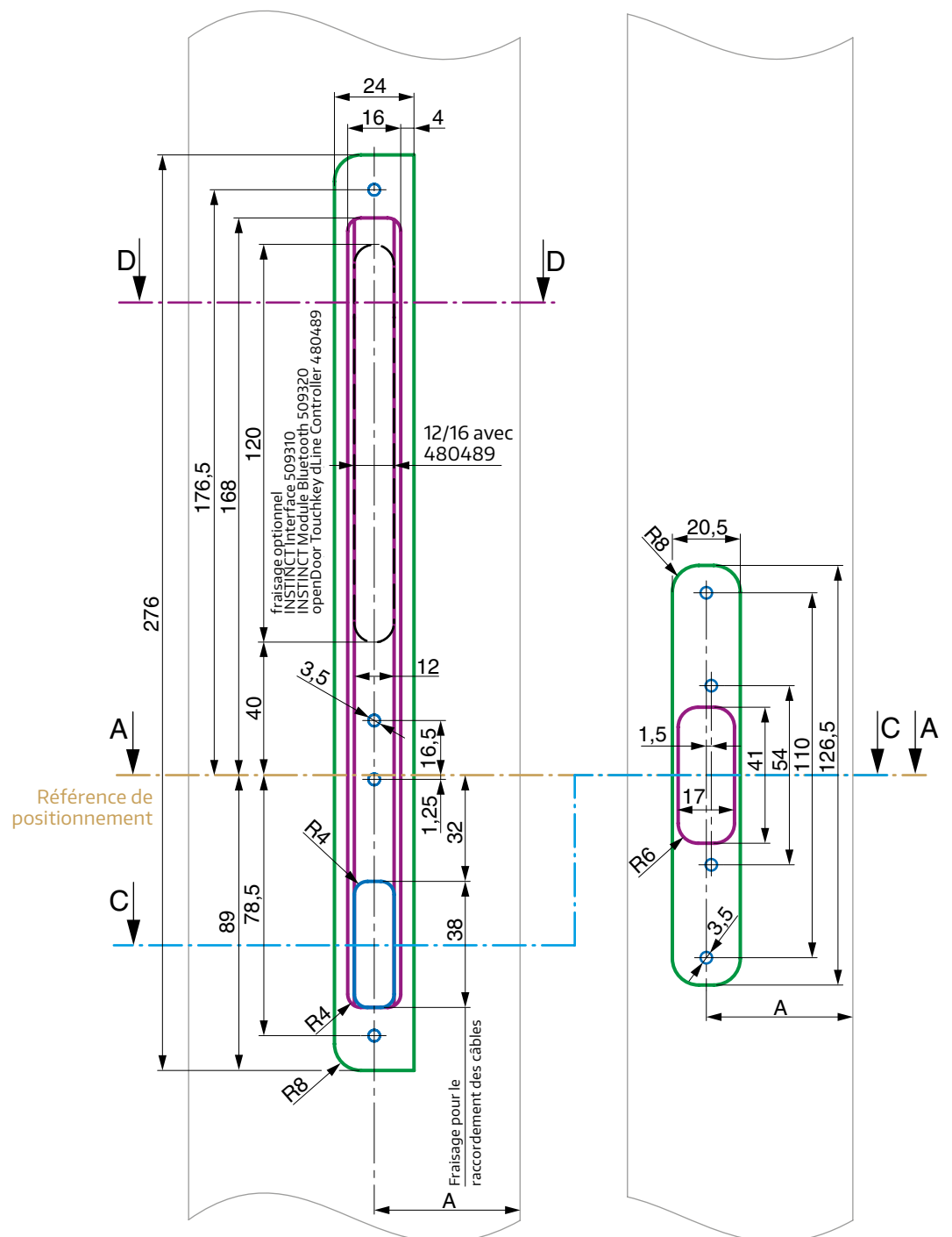
Profilé vantail (représentation simplifiée)
