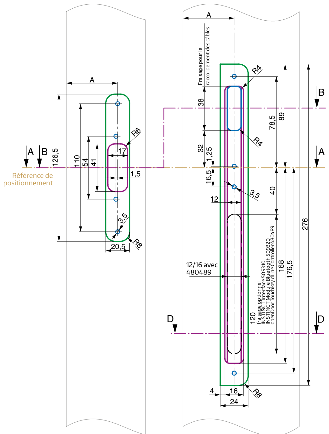
Profilé de dormant (représentation simplifiée)
