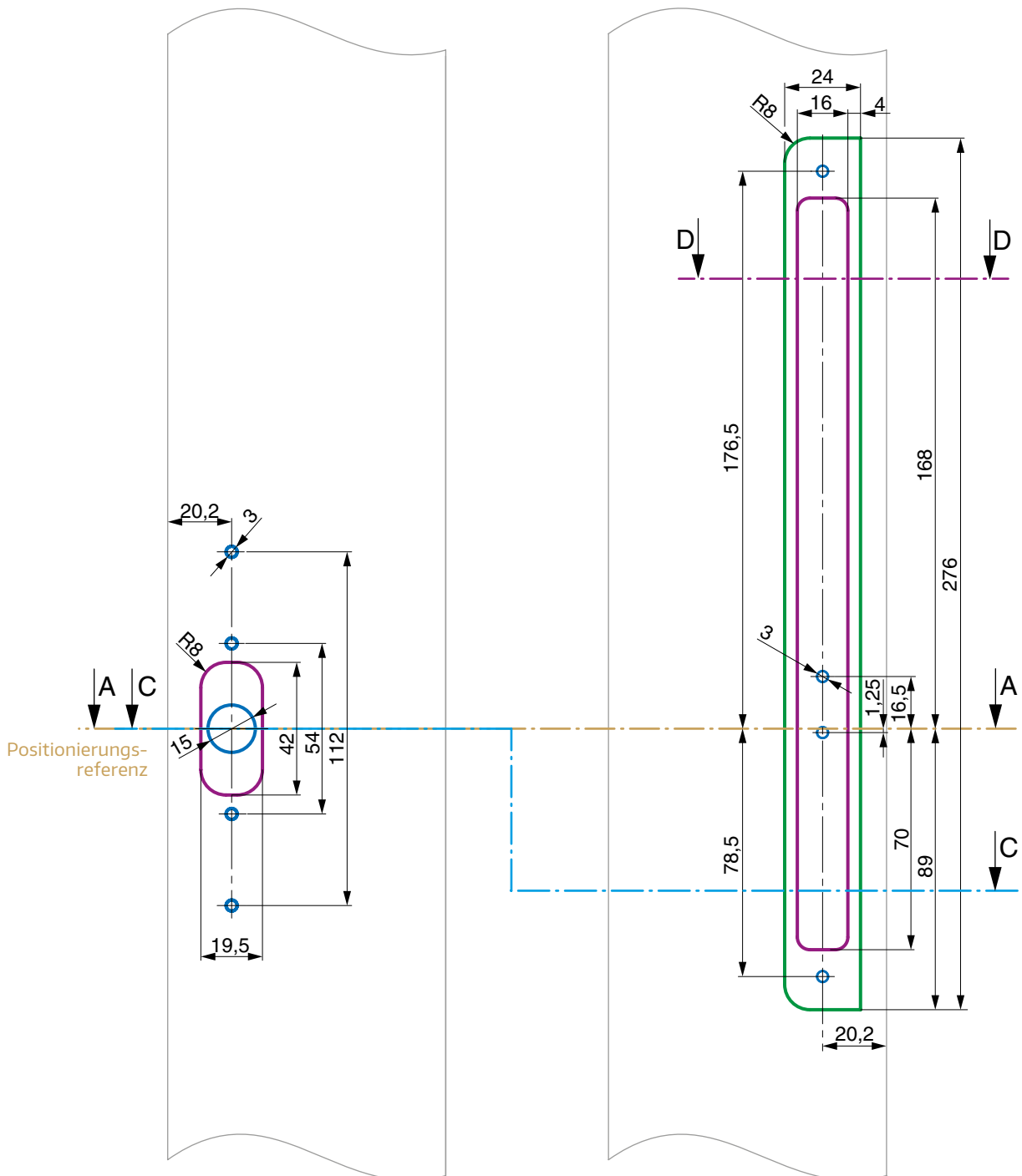
Flügelprofil (vereinfachte Darstellung)
