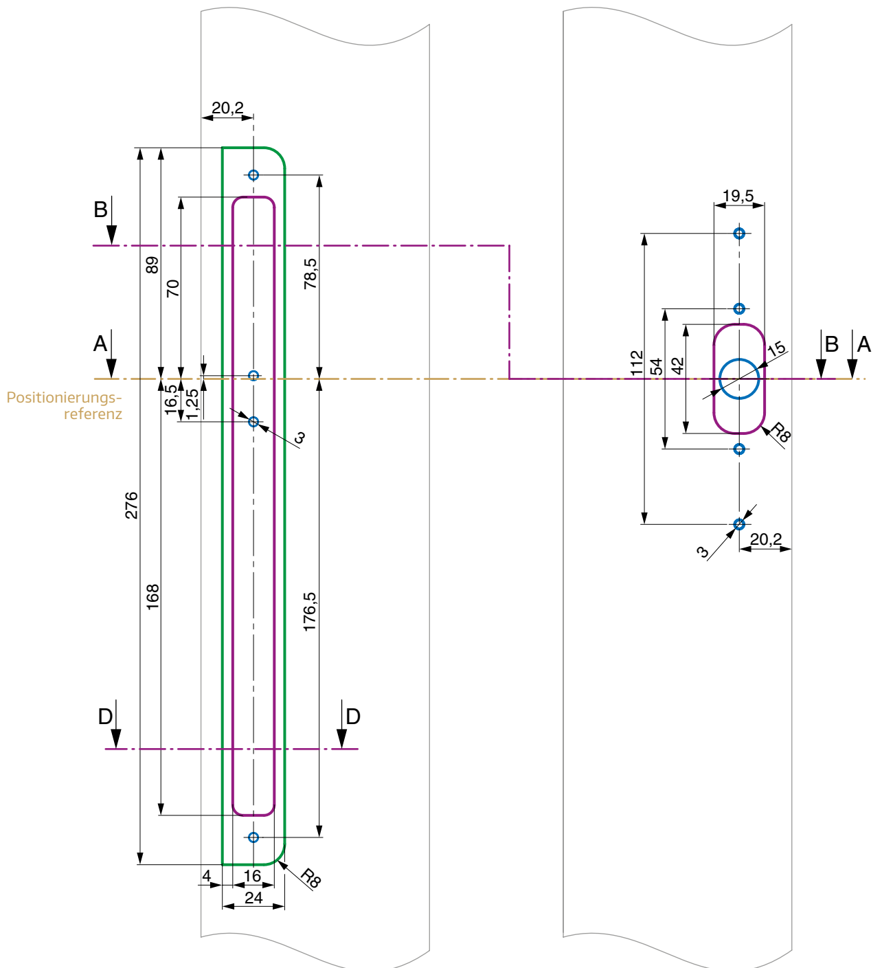
Rahmenprofil (vereinfachte Darstellung)
