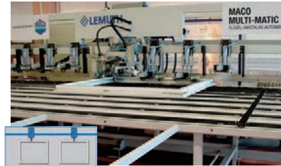
全机械自动化组装
