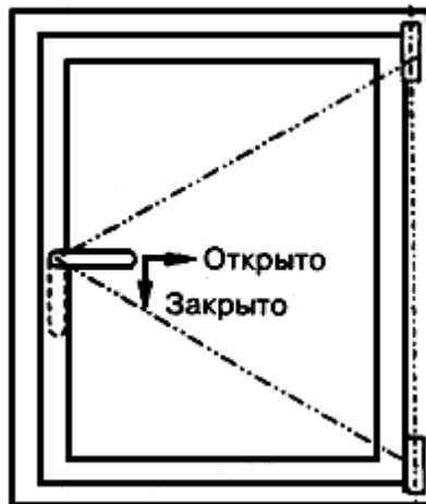
Рисунок А.1 – Поворотное устройство
