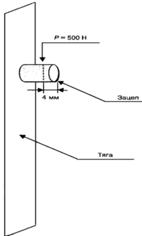
Рисунок Г.6 – Испытание крепления зацепа (см. 5.4.6)
